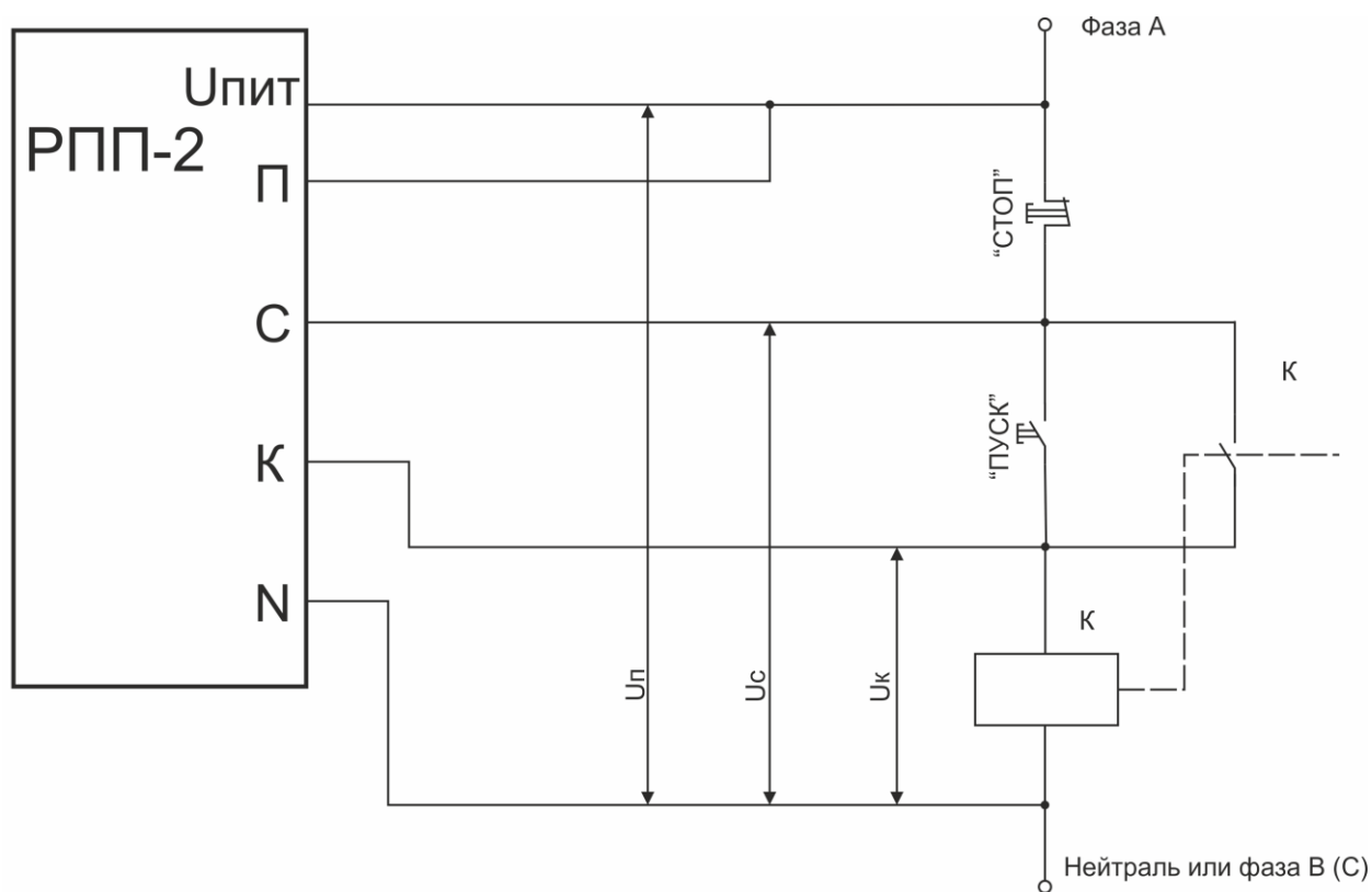
Рисунок 2 – Подключение реле к аппарату управления электродвигателем
