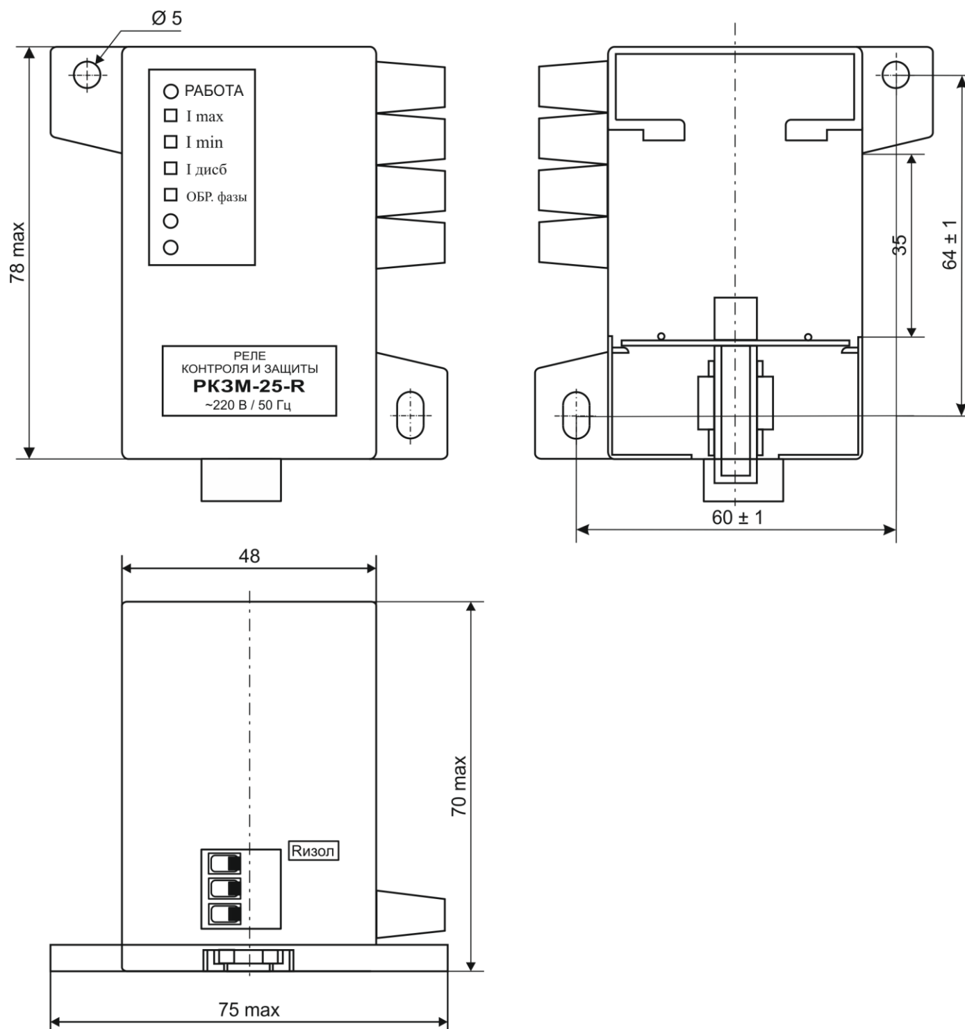
Рисунок 4 – Габаритные и установочные размеры реле
